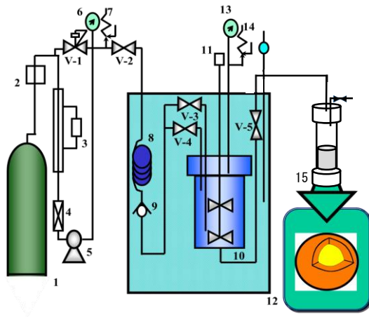
実験装置図
